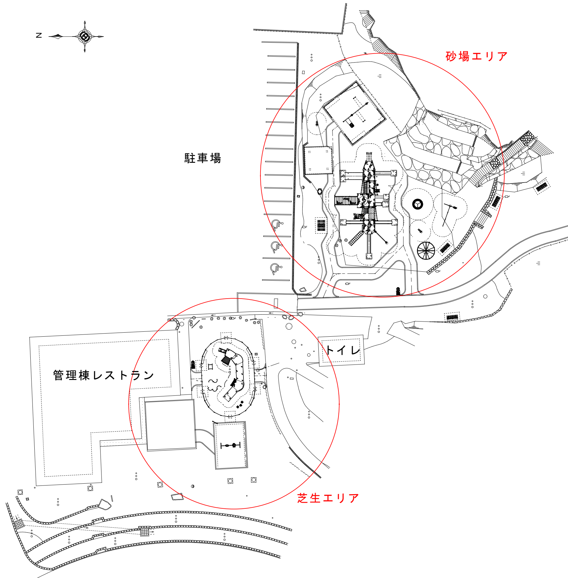
泊城公園平面図
