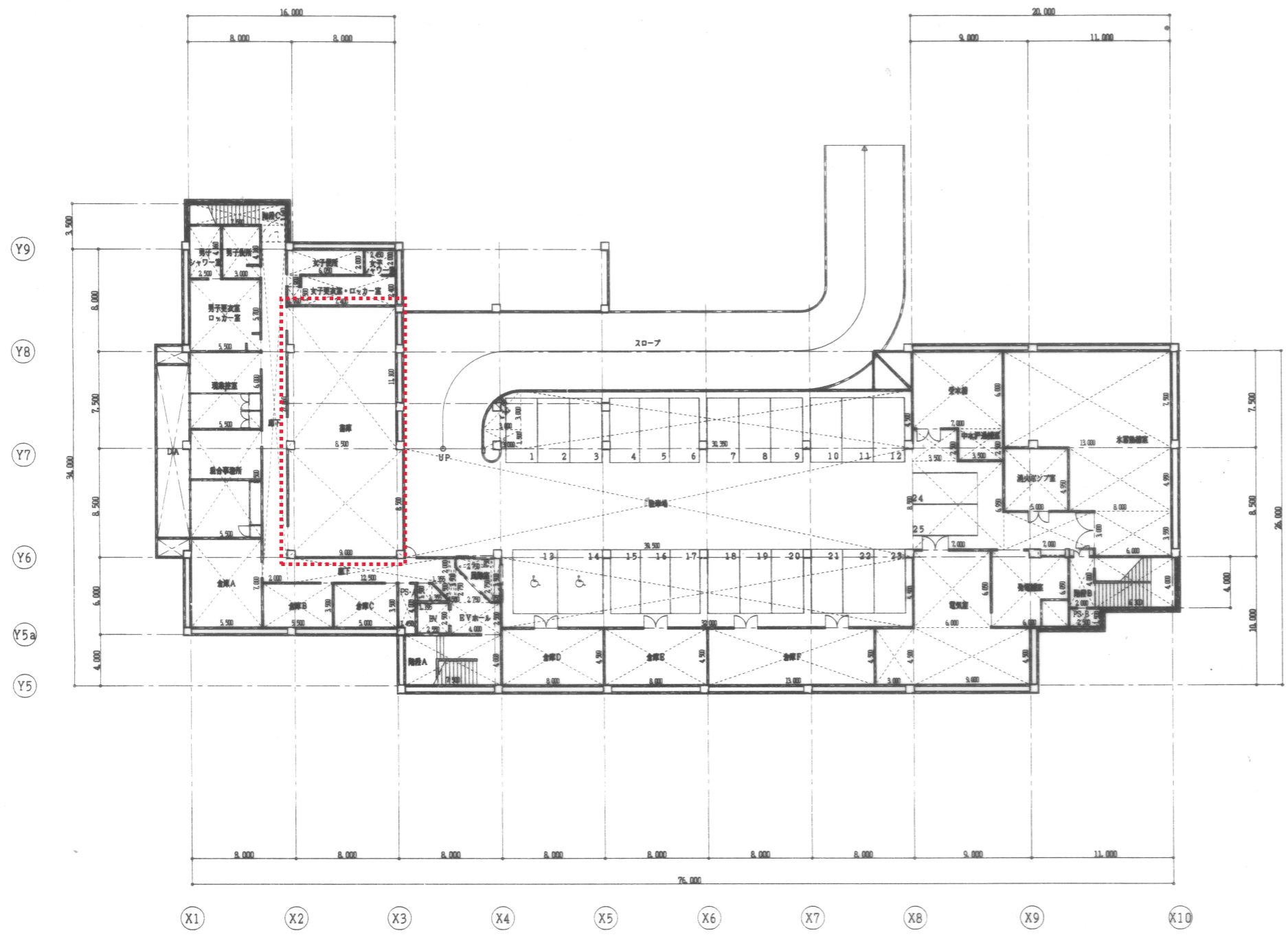
地階平面図 S=1:200
