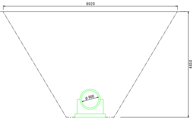
既設管撤去 断面図
