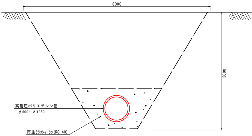
新設雨水管 断面図
