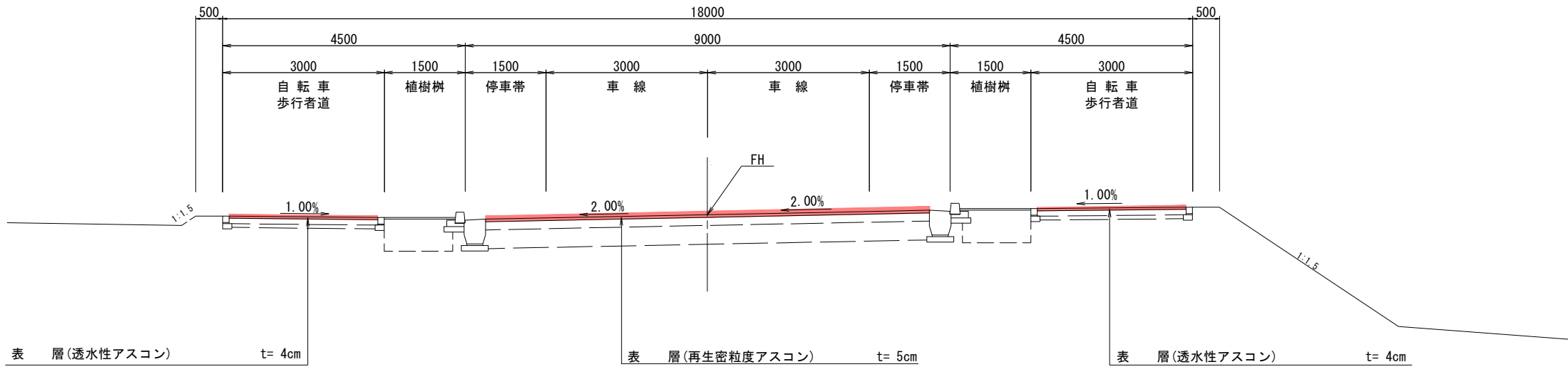
標準部 NO. 41付近 S=1/50
