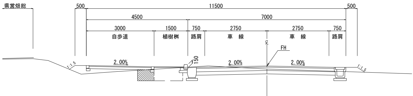
標準部 NO. 52～NO. 75付近 S=1/50 区画線のみ
